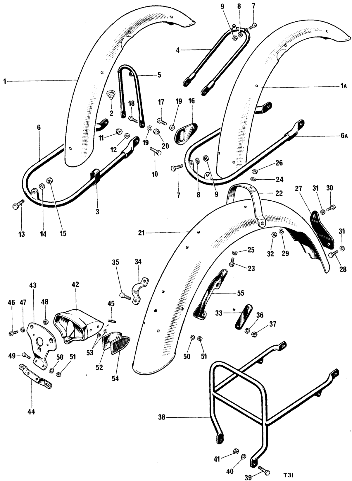
Fig. 28. MUDGUARDS (FENDERS)
