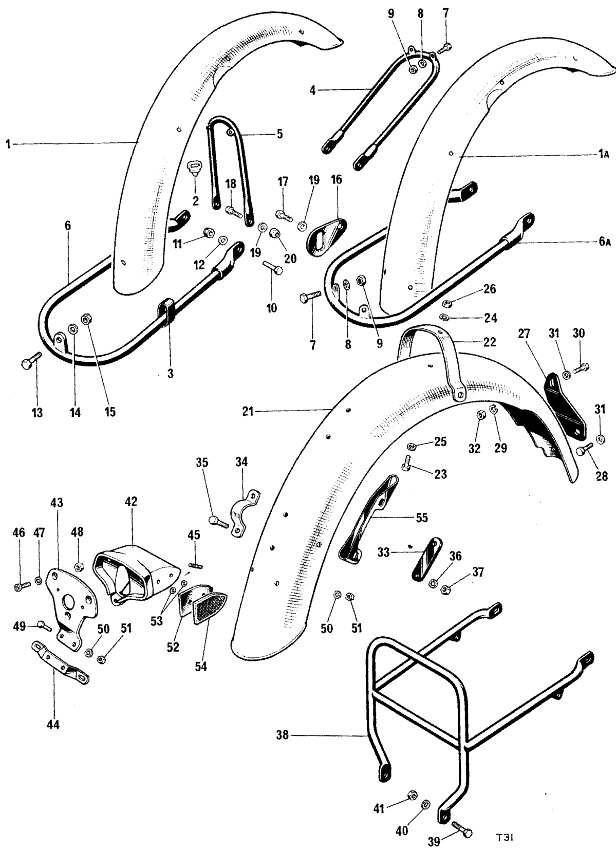
Fig. 29. MUDGUARDS (FENDERS)
