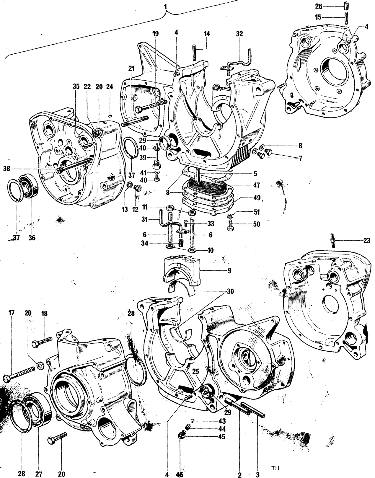
Fig. 2. CRANKCASES
