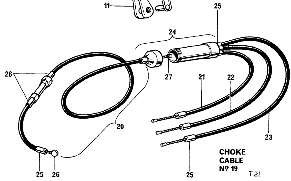
Fig. 31. CONTROL CABLES
